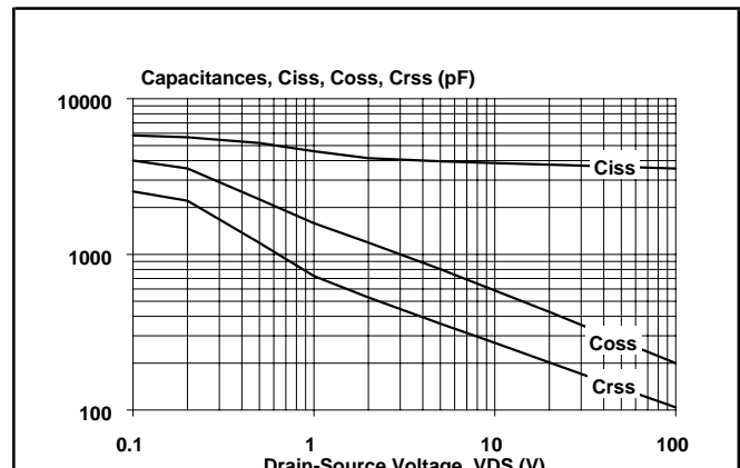
Fig. 12. Typical capacitances, C_{iss} , C_{oss} , C_{rss} .
